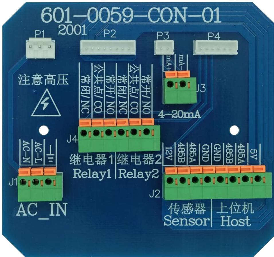
图 2.1 背板示意图
