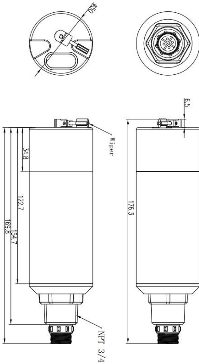
图 1-2 结构图
