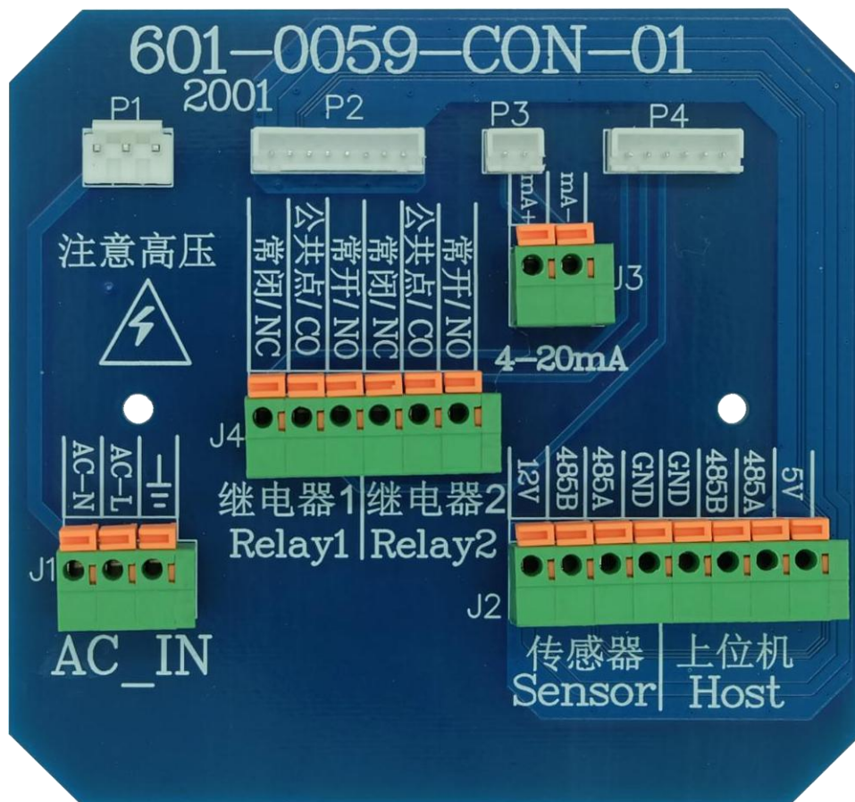
图 2.1 背板示意图
