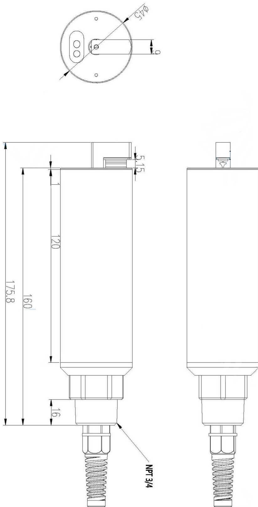
Y513-A 在线自清洁蓝绿藻传感器结构图
