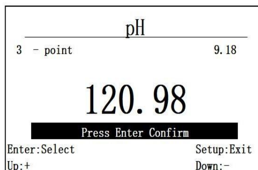
图 6.13.3 pH 的第三个校准点
