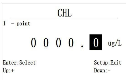
图 6.7.3.1 两点校准第一点校准值“0”
